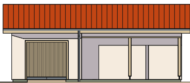
NORDOST-ANSICHT
